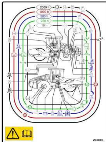
Esquema general de mantenimiento
